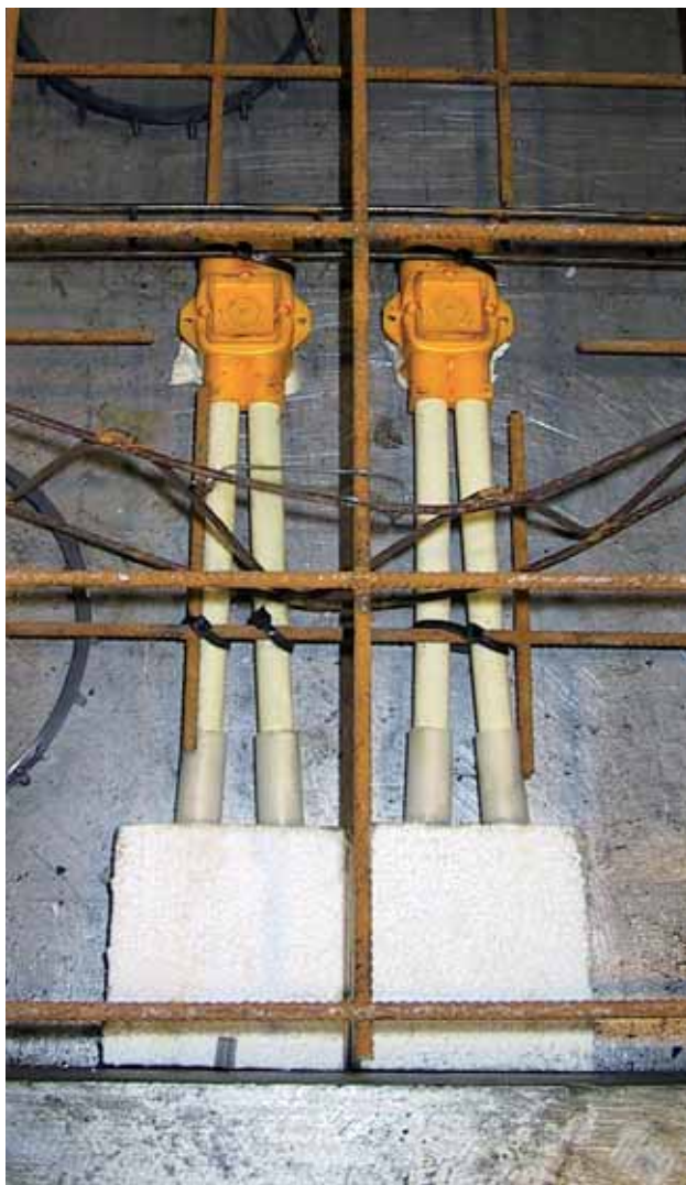
Figur 27. Udskæring i armeringsnet for el-dåser. 2 lodrette tråde er skåret over for at give plads til dåserne. Der er ikke skåret ud for rørene. Det kan – uanset dåsernes udformning – ikke undgås, at der må skæres tråde over for at skabe plads til dåserne.
