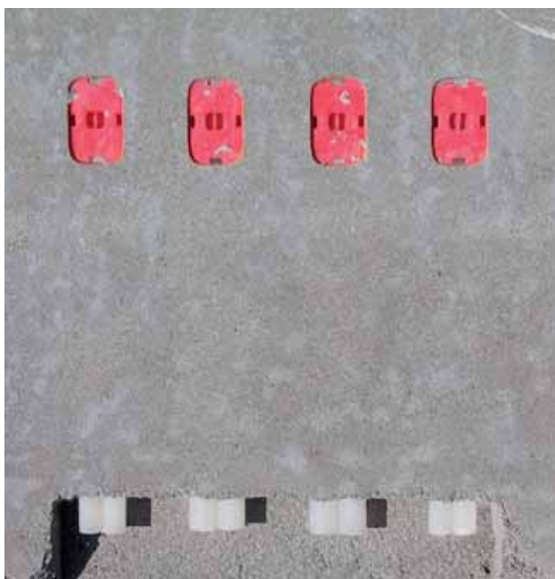
Figur 35. Det færdige resultat. 4 FUGA 1 1/2 M dåser (gl. type) indbygget i opsidens af et letklinkerbetonelement. Dåsernes indbyrdes placering er her sikret v.h.a. et patentbånd fastgjort med skruer til de enkelte dåser. Der er ingen vandret rørforbindelse mellem dåserne, al fremføring sker nedefra. Anvendes de nye FUGA dåser, kan der etableres en vandret forbindelse v.h.a. afstandsstykket LK nr. 504 N 1021. Dette gør det muligt at reducere antallet af lodrette rør. Man skal dog være opmærksom på, at afstandsstykket ikke giver mulighed for fuld omstøbning med letklinkerbeton, og der må påregnes en efterreparation af vægoverfladen mellem dåserne. Endelig skal det bemærkes, at vandrette dåsekombinationer reducerer væggenes tværsnit, hvilket kan have betydning for væggenes bæreevne.
