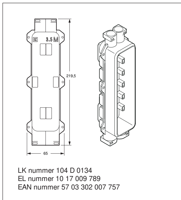
Figur 3. Gammel LK FUGA dåse 3½M
